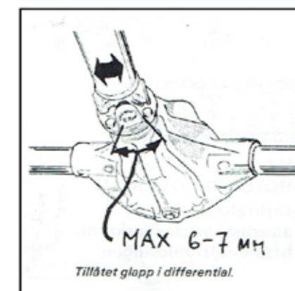
Fig. 52-7 Måling af slør i bagtøj
